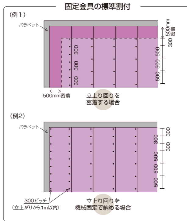
メルソーチ接合部の固定金具の位置
