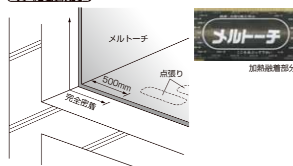
立上りからの納まり図
