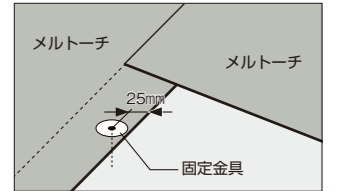
メルソーチ接合部の固定金具の位置
