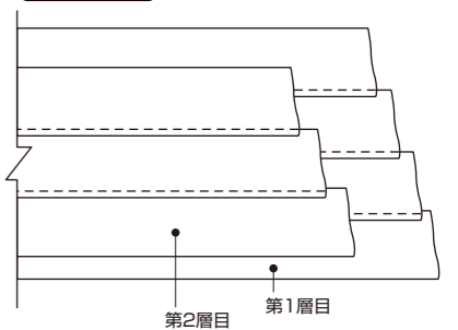
平場の納まり図
