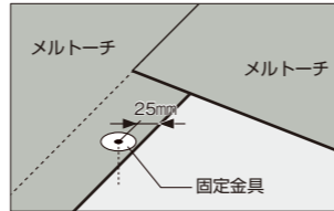
メルソーチ接合部の固定金具の位置
