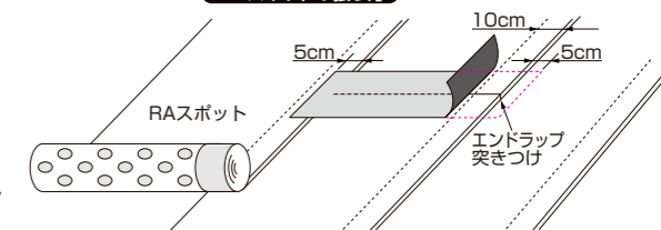
RAスポットの張り方
