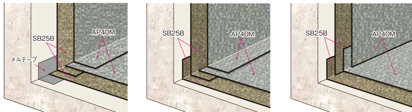
AS-T1・AS-T3・AS-T4仕様
